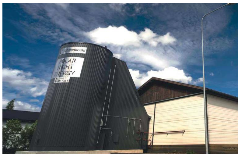
Vysokoteplotní pískové úložiště – dlouhodobá akumulace tepla (léto/zima)
